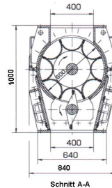
8-Kammer Zwangsräumssystem
